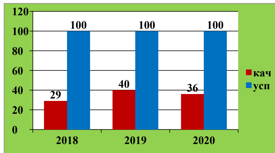
Физика.
