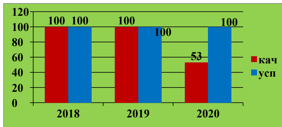
Физика.
